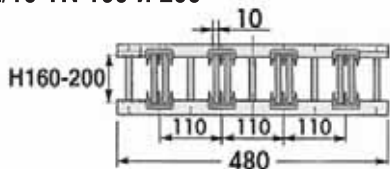
Типы UBS 2/10 TN 160 и 200
